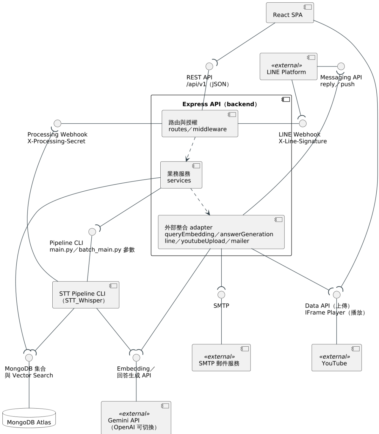
圖 7-3-1 系統元件圖
