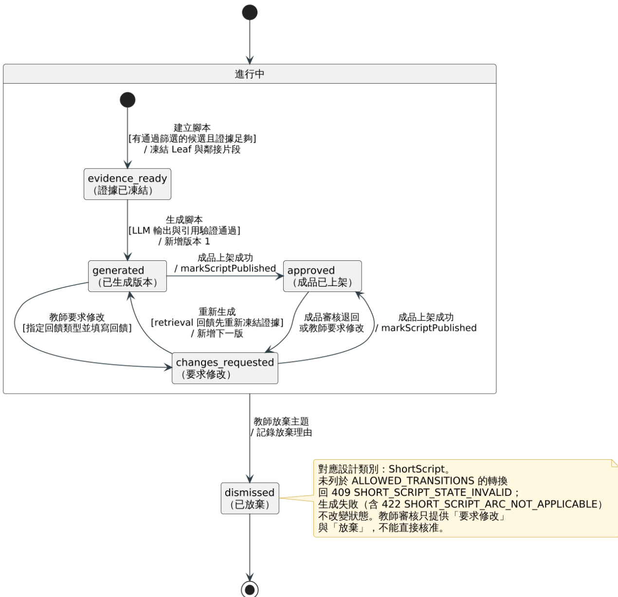
圖 7-4-7 短影音脚本状态机图
