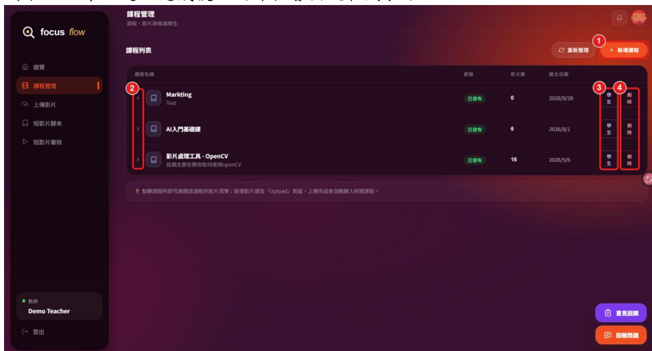
圖 12-4-2 課程列表
