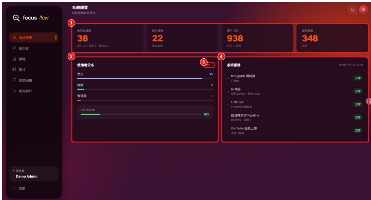
圖 12-5-1 系統總覽
