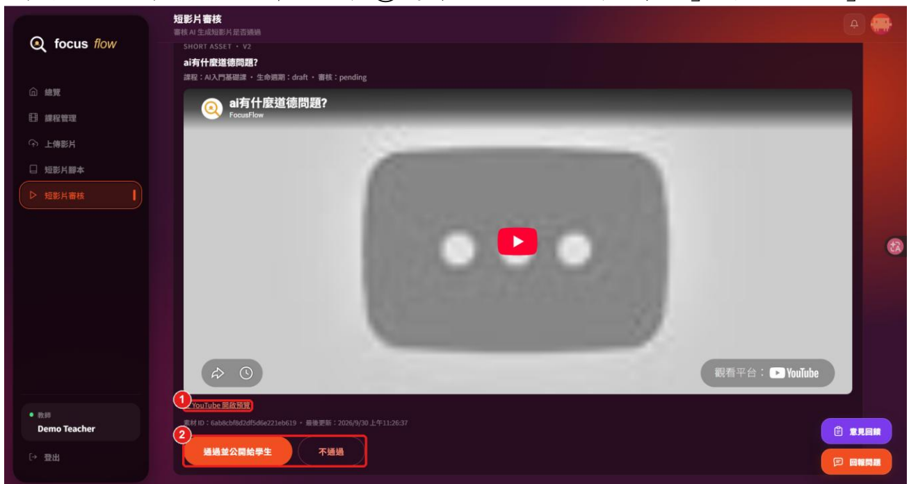
圖 12-4-12 審核決定
