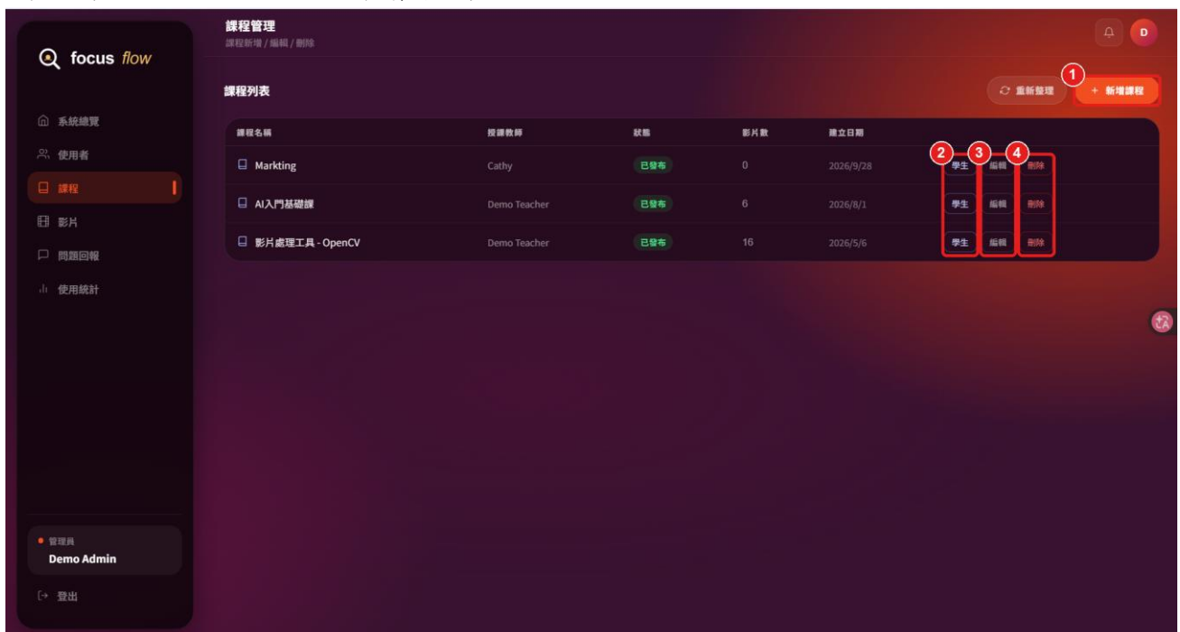
圖 12-5-3 課程管理
