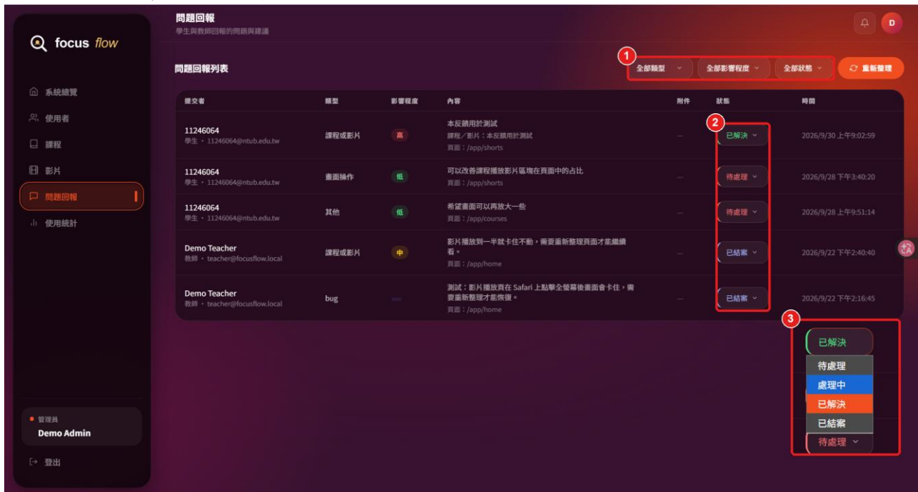
圖 12-5-6 問題回報
