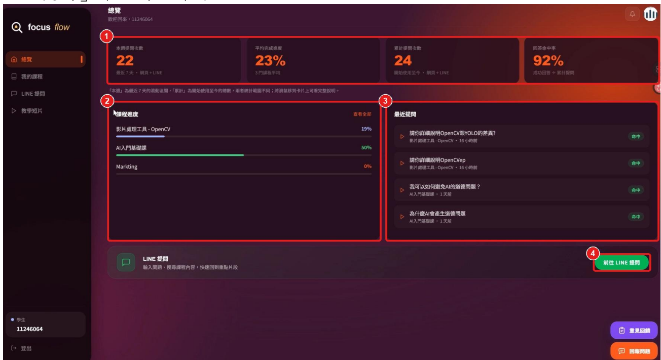
圖 12-3-1 學生總覽
