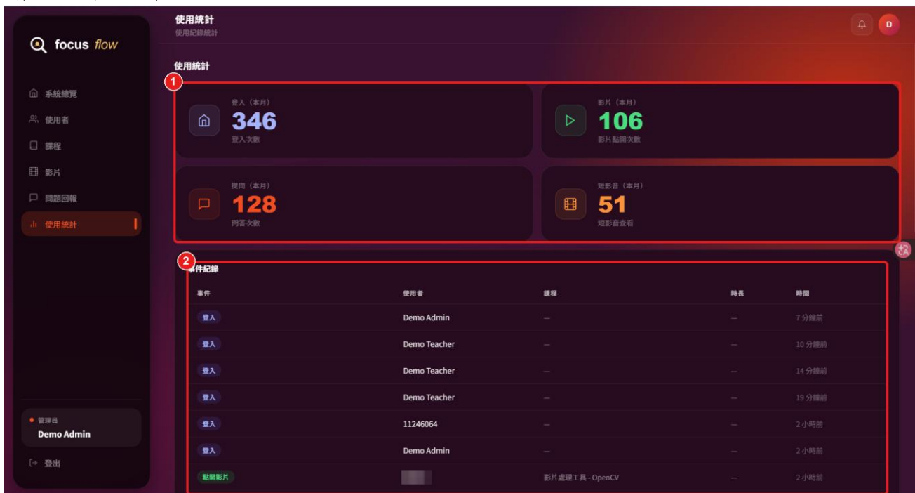
圖 12-5-7 使用統計
