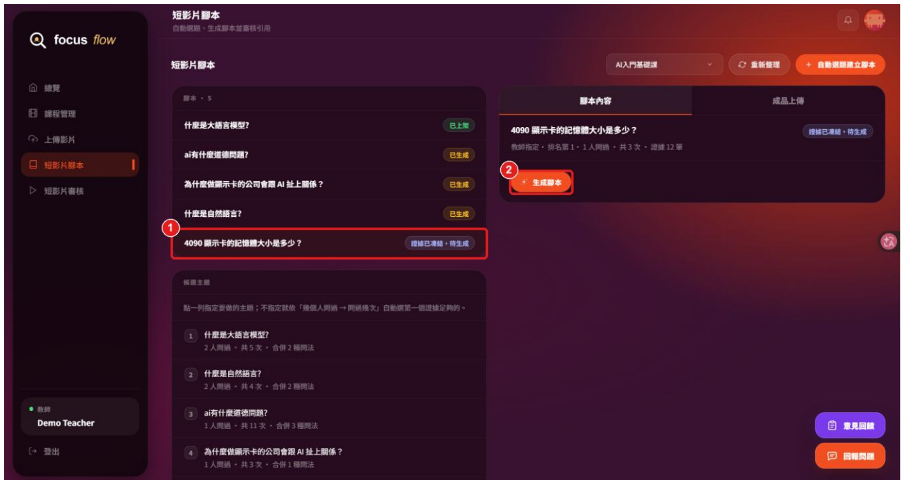
圖 12-4-8 建立新腳本
