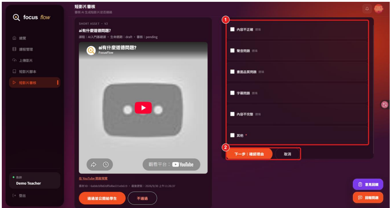
圖 12-4-13 不通過理由
